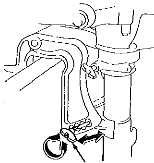
tilttipuikko ja siipimutteri
